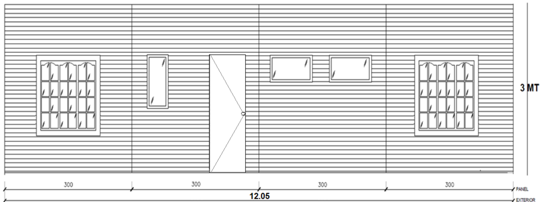
ELEVACIÓN POSTERIOR ESCALA 1:50
